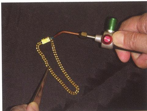
貴金属のロー付け作業
