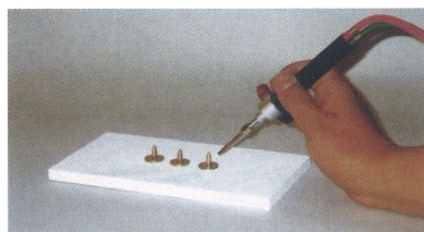
▲リトルトーチによる銀ろう加熱作業 ▲ディスペンサによる銀ろう供給
